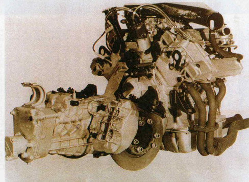
Groupe moto-propulseur (extrait du dossier de présentation au concessionnaire en mai 1970)
